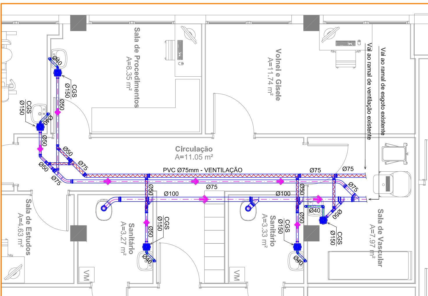
PLANTA BAIXA - ESGOTO
