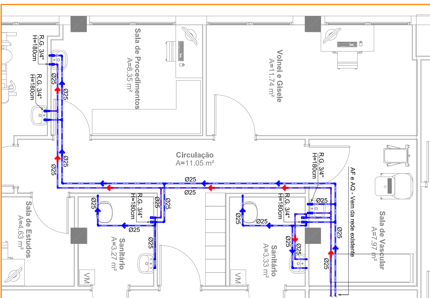
PLANTA BAIXA - AGUA ESCALA 1:50
